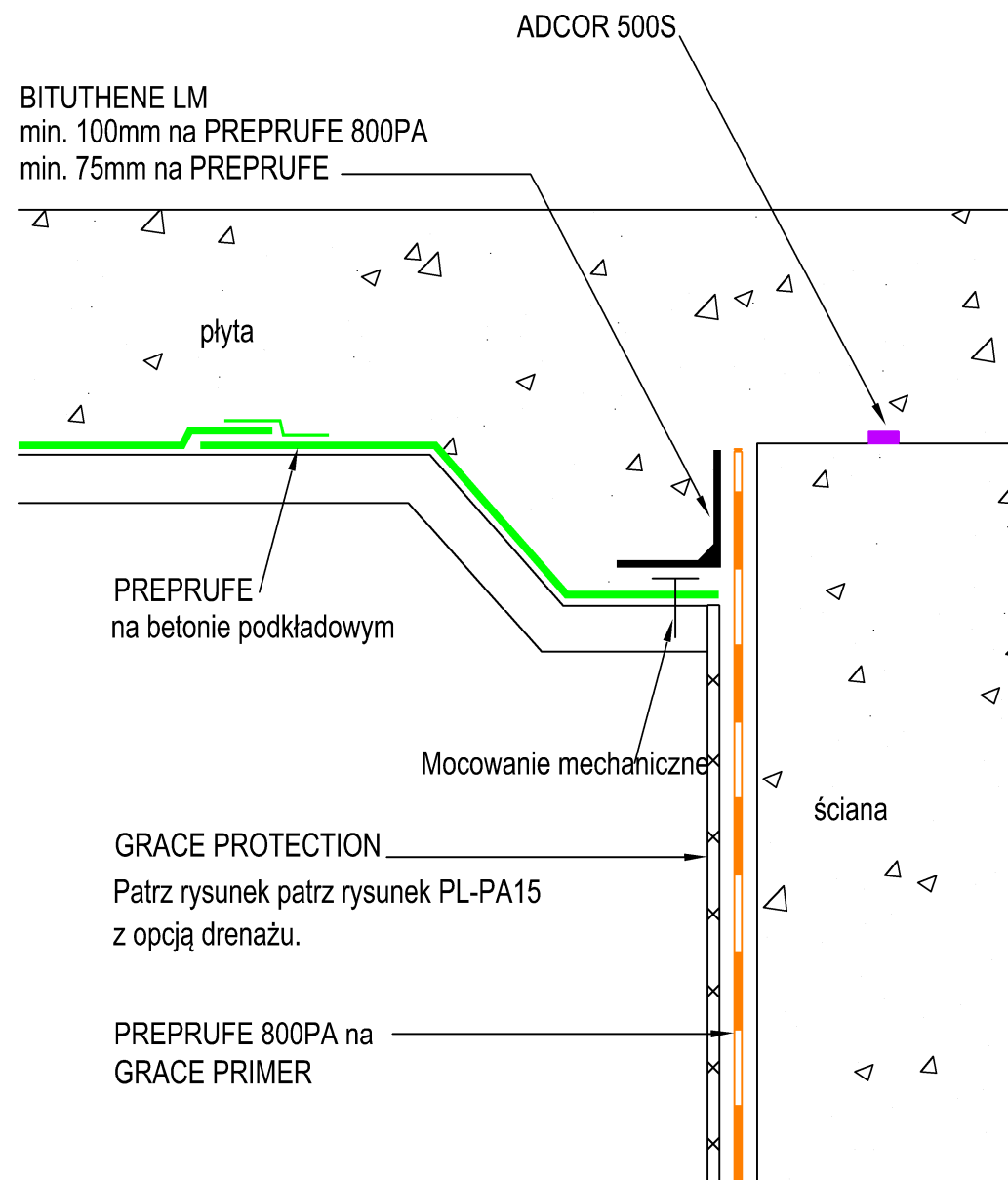
DETAL POŁĄCZENIA ŚCIANY W GÓRNYM POZIOME PŁYTY SEKCJA
